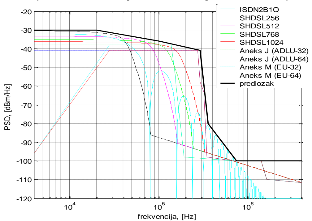
Slika 5.7.6 Frekvencijski predložak za odlazni smjer prijensa (duge pretplatničke linije) za ADSL preko ISDN (aneks B).
