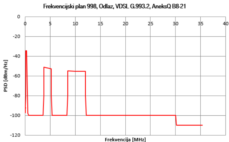
Slika 5.7.4 Frekvencijski predložak za odlazni smjer prijenosa za VDSL2, frekvencijski plan 998, B8-21
